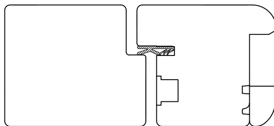
Sez C-C BILICO NODO AL SOTTO DEL CENTRALE
