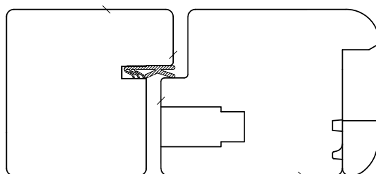
Sez B-B BILICO NODO AL SOPRA DEL CENTRALE
